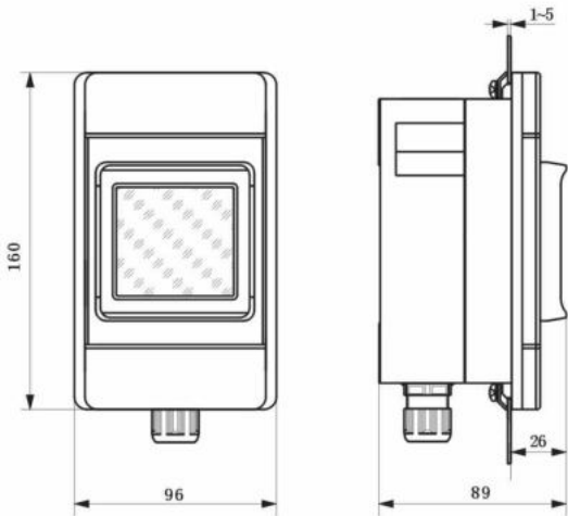
外形尺寸 Outline dimensions:
