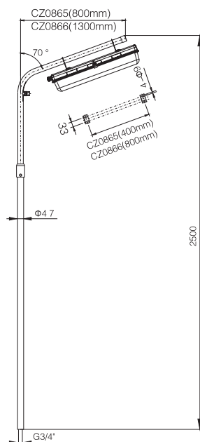
护栏式安装
