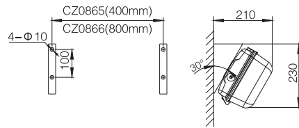
吸壁式安装
