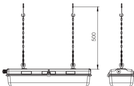
吊链式安装
