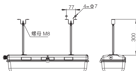
吊杆式安装
