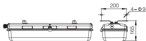
吸顶式安装
